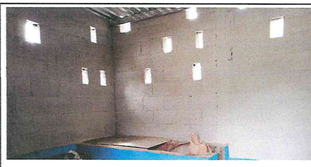
Foto 6: sellado de base de chimenea que se colocara en la parte exterior de la cocina para que salga el humo y no se retenga en el interior de la misma
